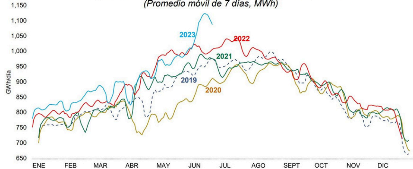
Energía consumida en el Sistema Eléctrico Nacional 2019-2023 (Promedio móvil de 7 días, MWh)
