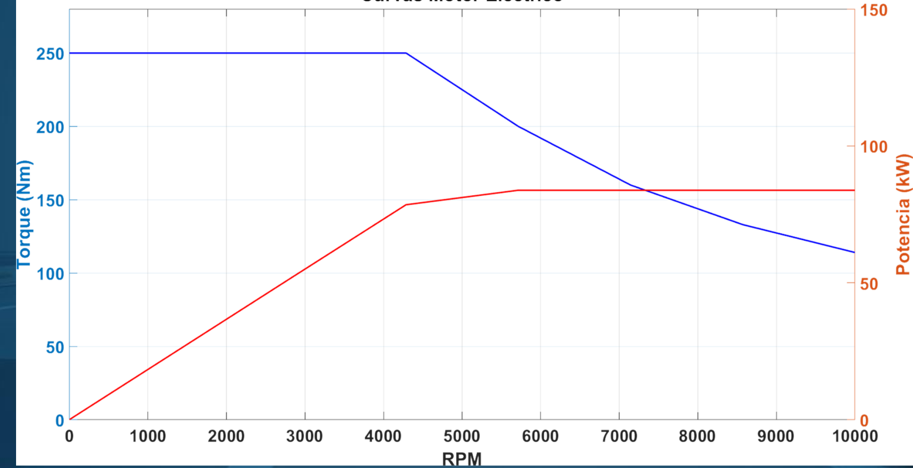
Curvas Motor Eléctrico
