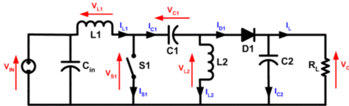
CONVERTIDOR SEPIC
