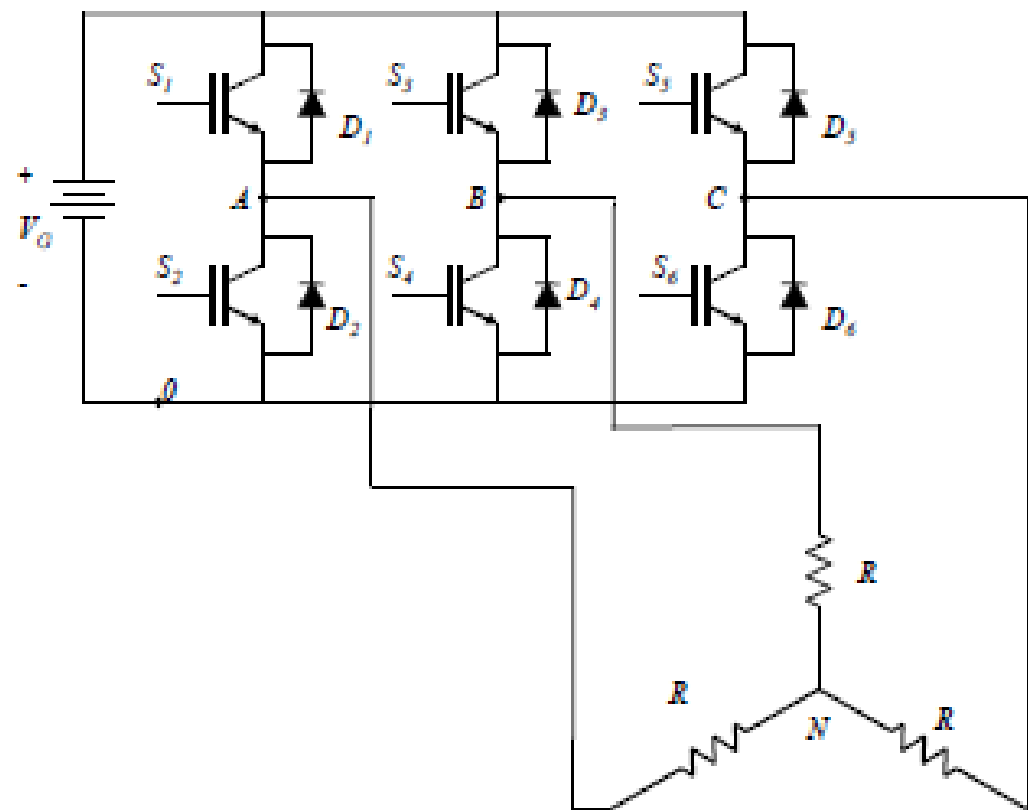
INVERSOR TRIFÁSICO
