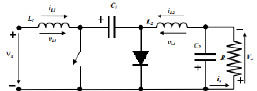
CONVERTIDOR CUK
