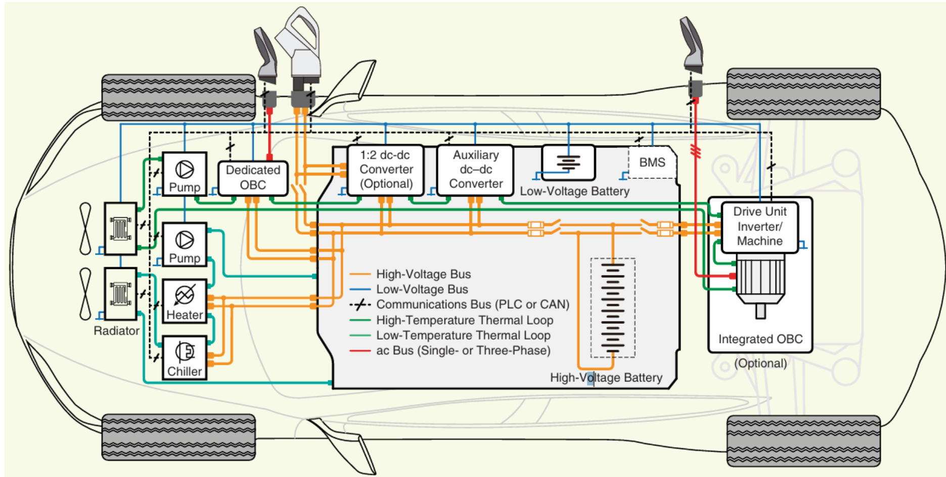
Diagrama electromecánico de un vehículo Eléctrico con carga rápida de DC.
