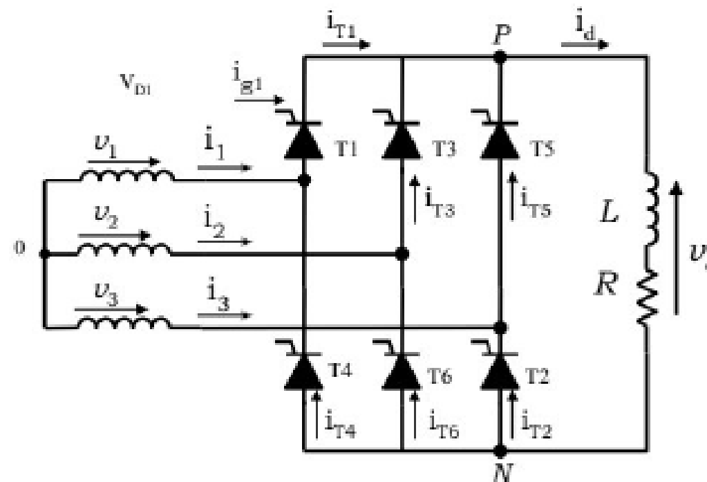
RECTIFICADOR CONTROLADO TRIFÁSICO
