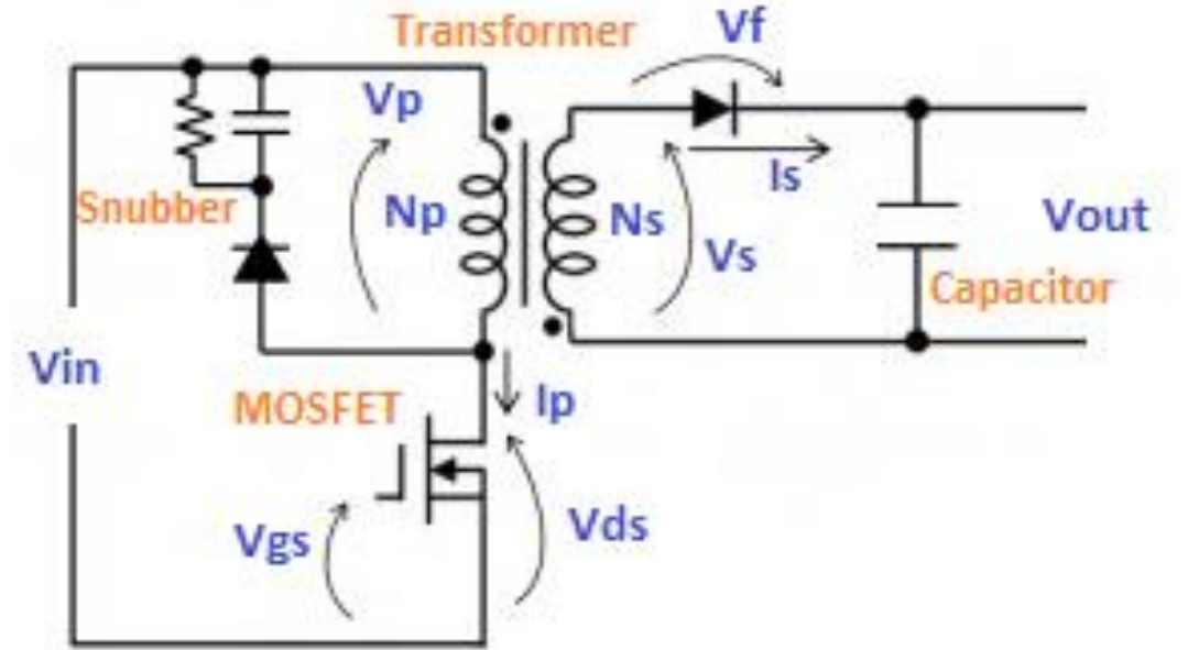
CONVERTIDOR FLYBACK
