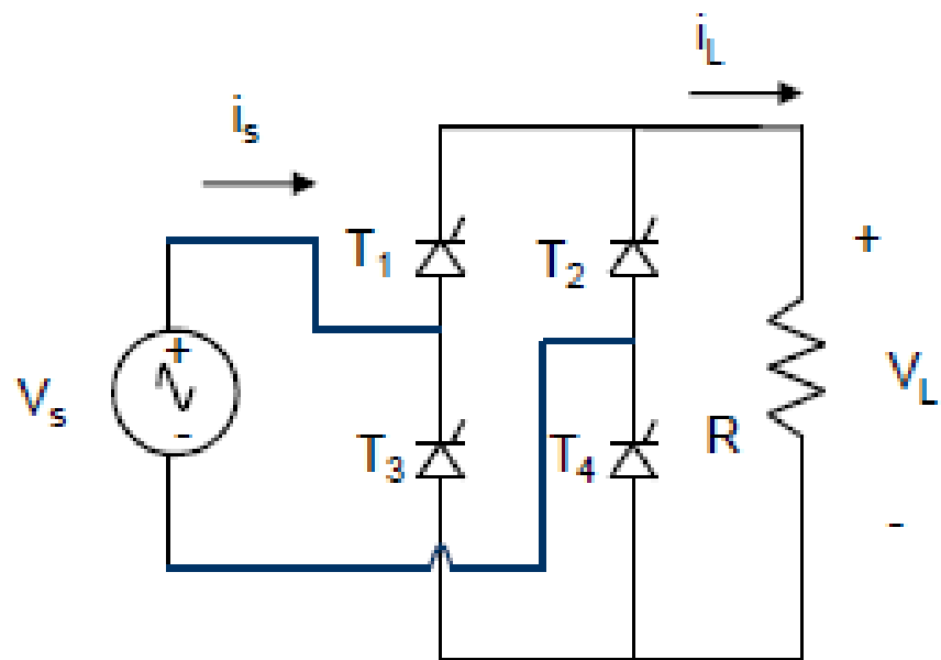
RECTIFICADOR CONTROLADO DE PUENTE COMPLETO
