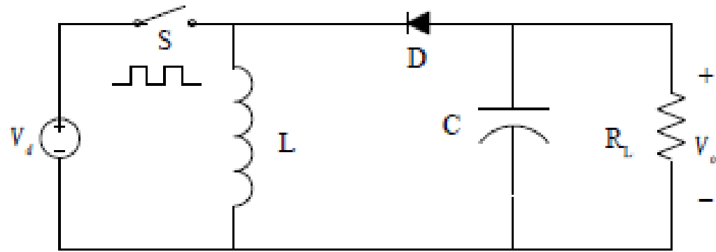
CONVERTIDOR REDUCTOR - ELEVADOR
