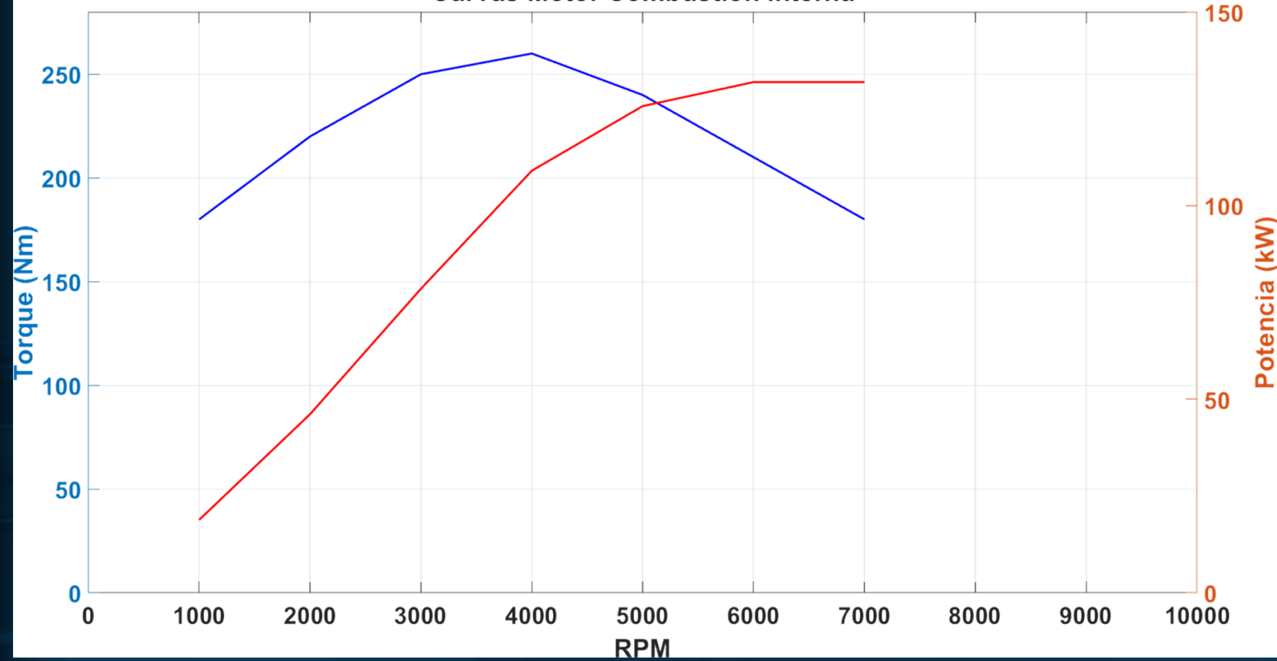
Curvas Motor Combustión Interna
