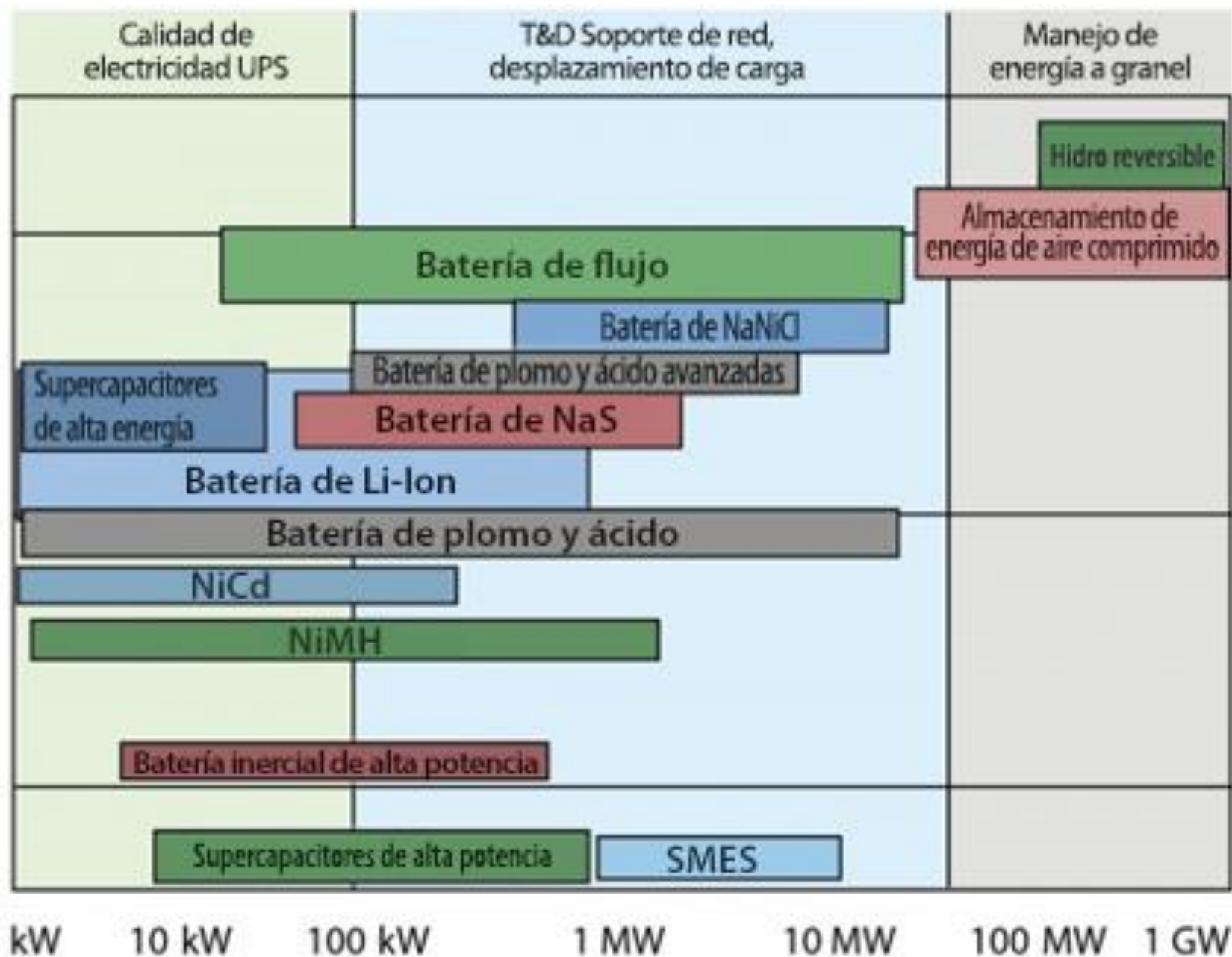
Clasificación de sistemas de energía, tamaño del módulo
