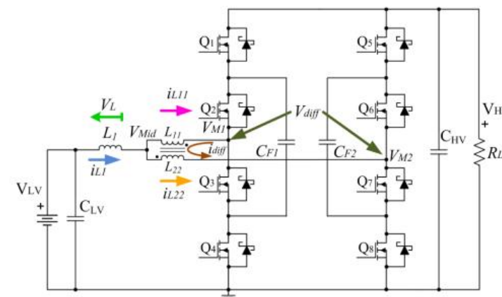
Convertidor DC-DC dual en fases intercaladas de tres niveles con Capacitor Flotante (FC)
